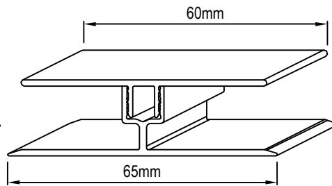
ALUMINUM H-MOLD
