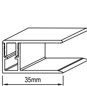
ALUMINUM J-MOLD
